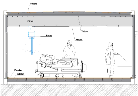
Coupe longitudinale
